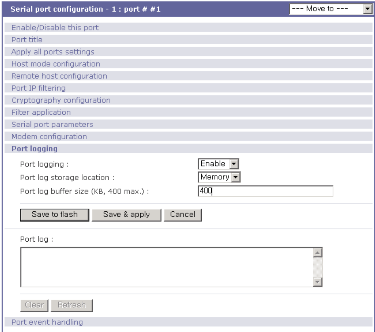
그림 4-17 Port logging configuration
