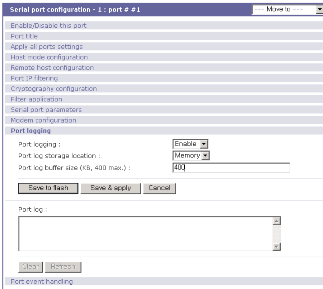
그림 4-17 Port logging configuration
