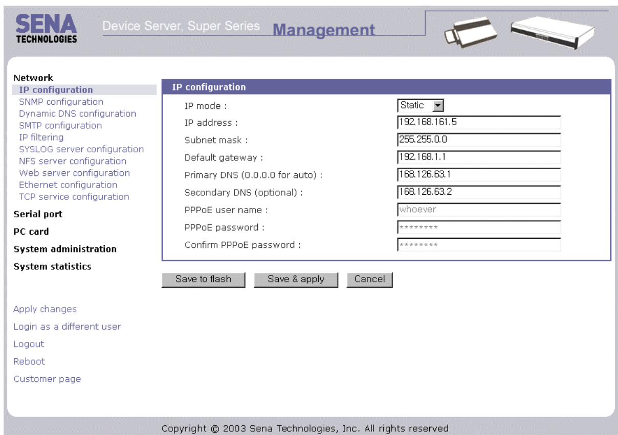
그림 2-18 Super Series 웹 관리 화면
