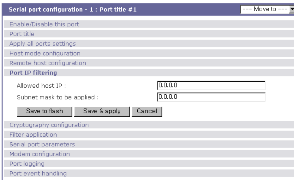
그림 4-9 Port IP filtering for serial ports
