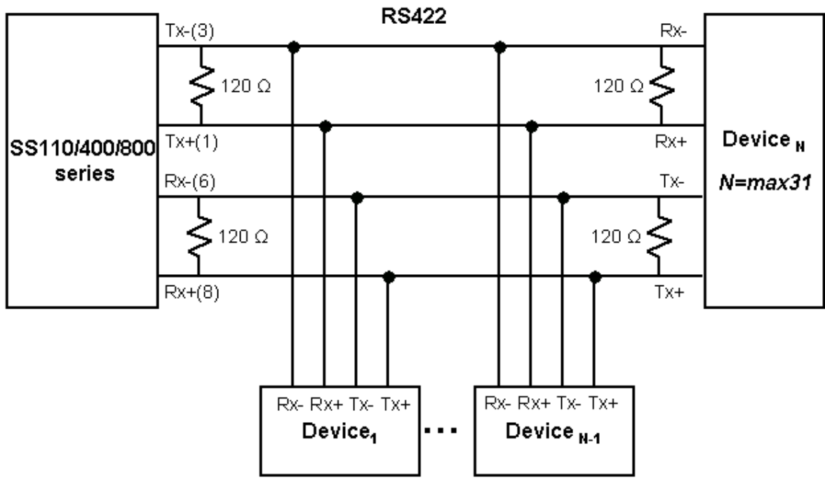
그림 A-9 SS110/400/800용 RS422 시리얼 배선도 RS422
