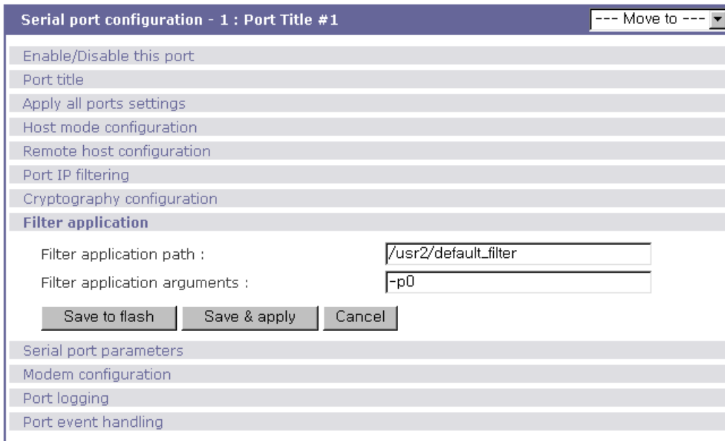
그림 4-14 필터 애플리케이션
