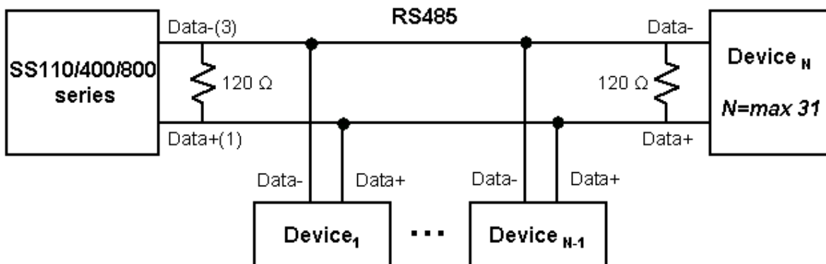
그림 A-8 SS110/400/800용 RS485 시리얼 배선도
