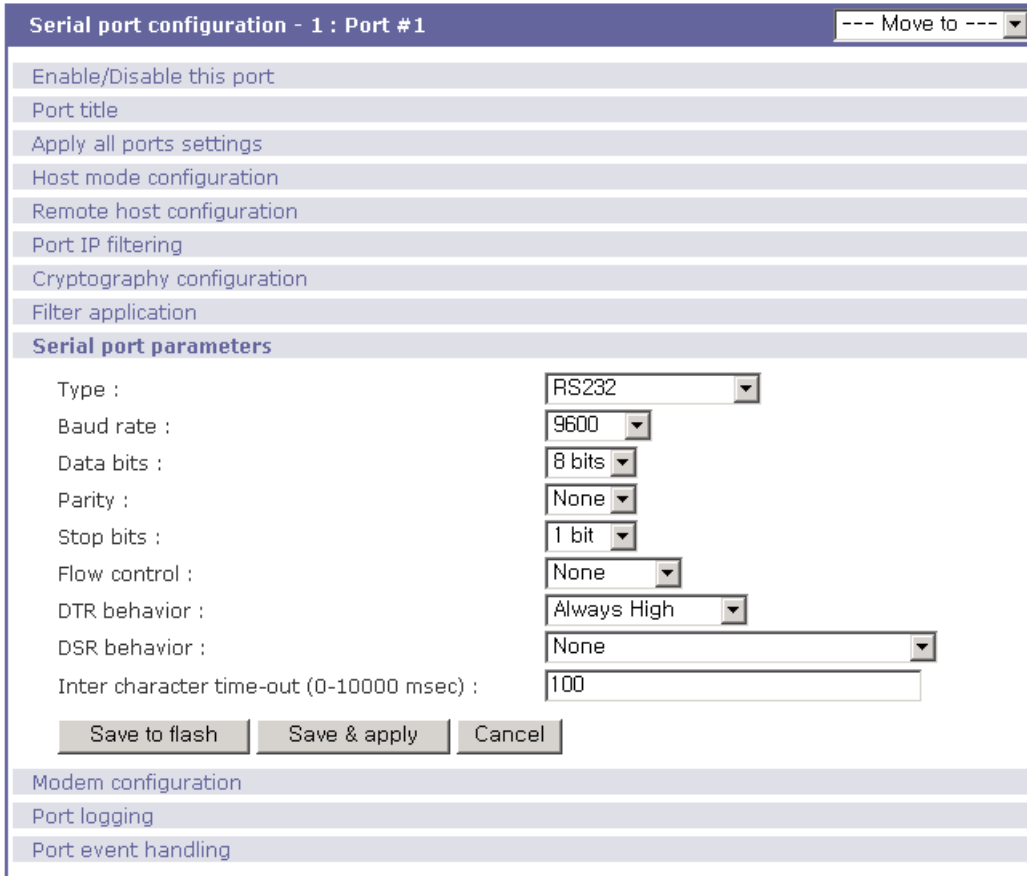
그림 4-15 UART 구성
