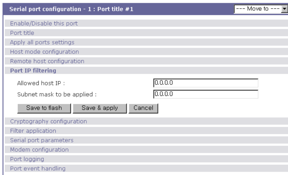
그림 4-9 Port IP filtering for serial ports
