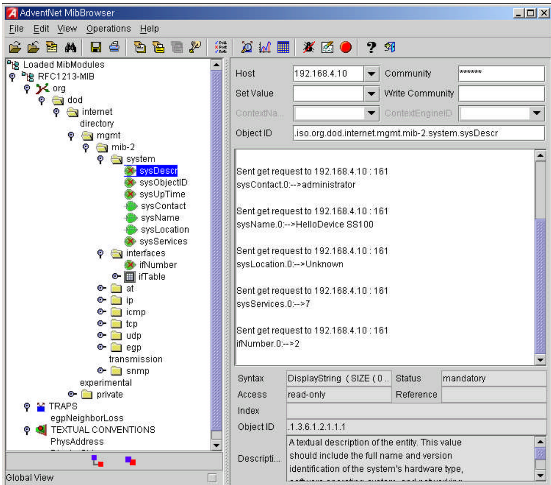
그림 3-3 SNMP 브라우저를 사용한 Super Series SNMP 에이전트의 MIB-II OID 브라우징 (AdventNet MIB브라우저)
