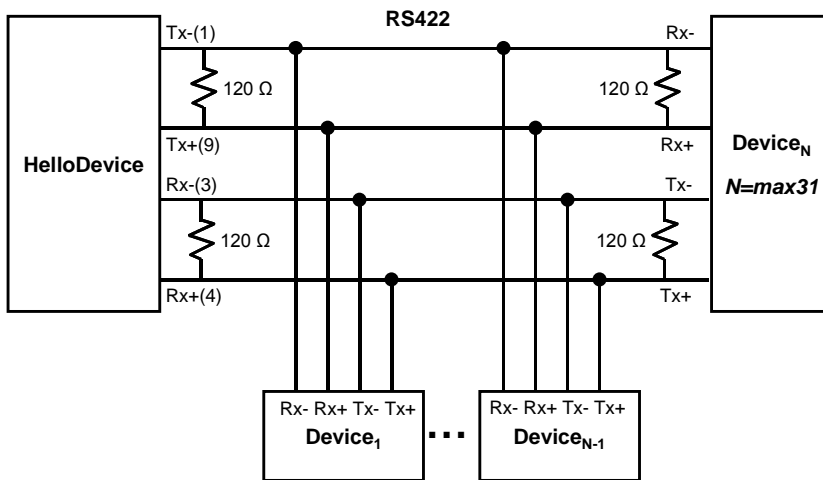
그림 A-7 RS422 시리얼 배선도(SS100용)
