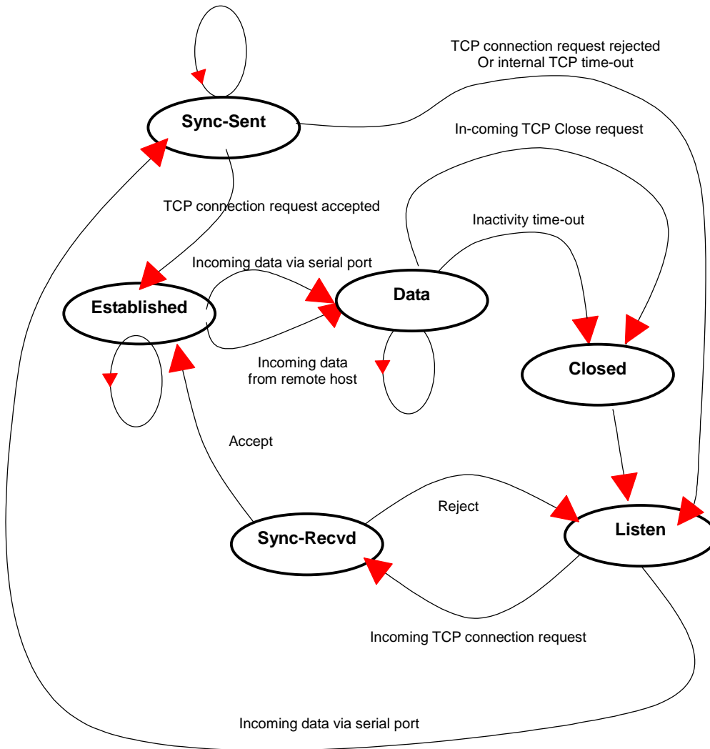
그림 4-6 TCP모드의 상태전이도
