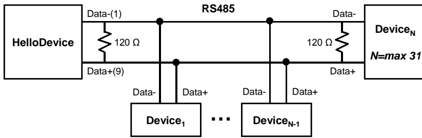
그림 A-6 RS485 시리얼 배선도(SS100용)
