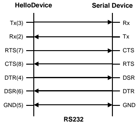
그림 A-5 RS232 시리얼 배선도(SS100용)
