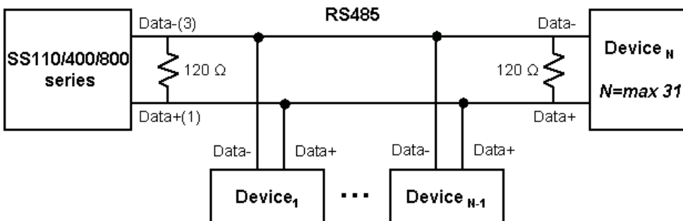
그림 A-8 SS110/400/800용 RS485 시리얼 배선도
