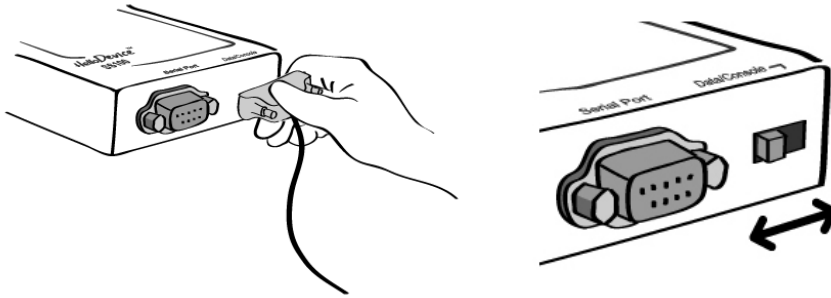
그림 2-12 SS100에 시스템 콘솔 케이블을 연결하기
