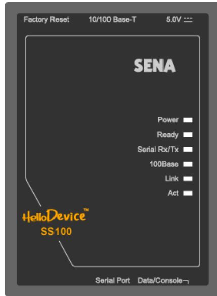
그림 2-1 SS100의 패널 레이아웃
