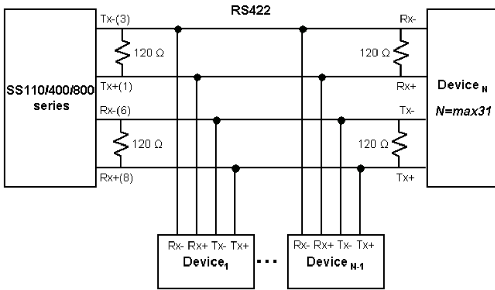
그림 A-9 SS110/400/800용 RS422 시리얼 배선도 RS422
