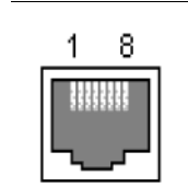
그림 A-1. RJ45 커넥터의 핀 배치
