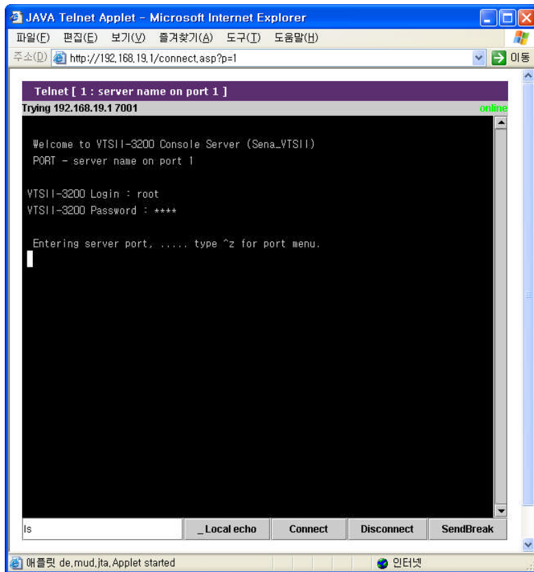
그림 4-39 Port number로 시리얼 포트에 직접 연결
