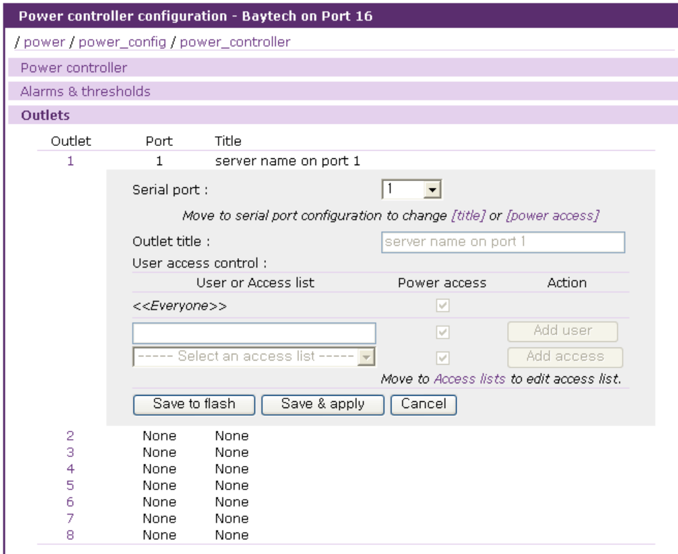
그림 6-6 파워 컨트롤러 유닛 설정 - 시리얼 포트에 연결된 아웃렛 설정
