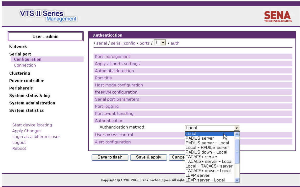
그림 4-22 시리얼 포트에 대한 인증 옵션
