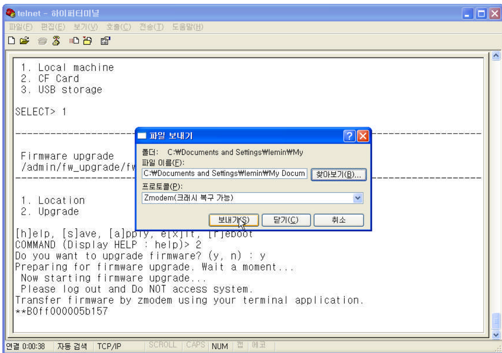
그림 9-13. Zmodem을 이용한 firmware 파일 전송 (Hyper Terminal)
