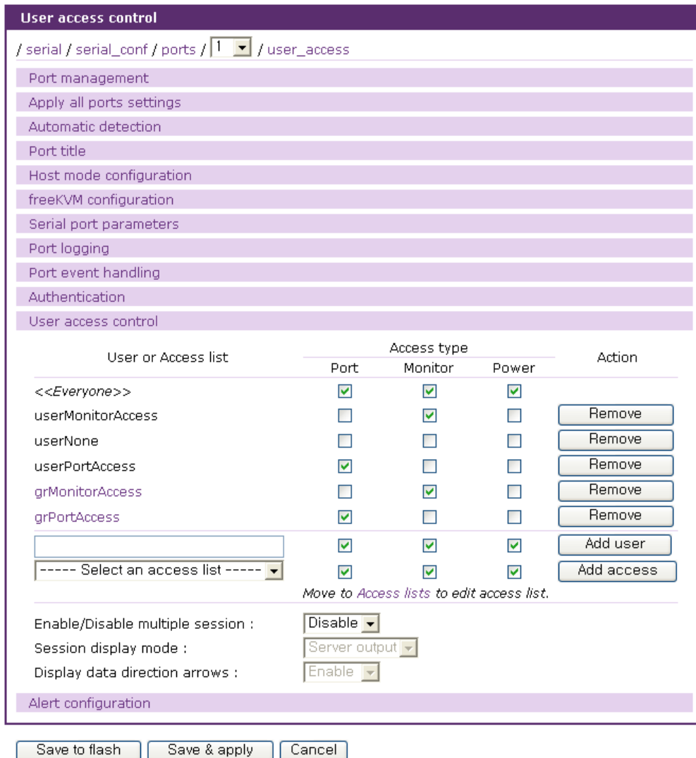
그림 4-24 시리얼 포트에 대한 액세스 제어 설정
