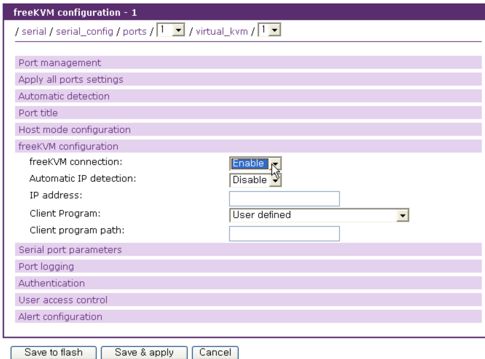
그림 4-14 freeKVM 세부 설정
