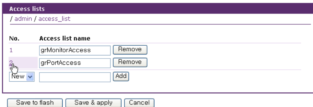
그림 9-3. 액세스 리스트 - 액세스 리스트 관리
