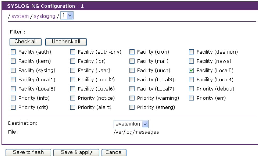
그림 8-4 SYSLOG-NG 세부 설정 화면
