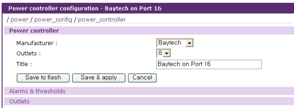
그림 6-2 파워 컨트롤러 유닛 설정 – power controller 탭
