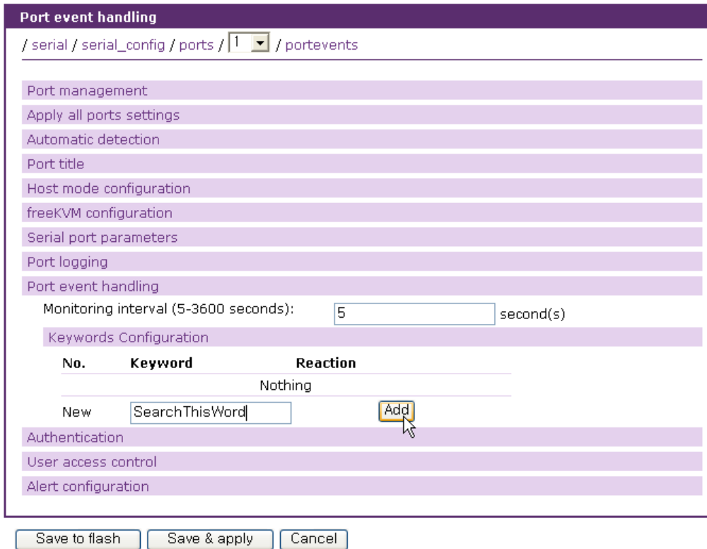
그림 4-18 포트 이벤트 핸들링 - 키워드 등록
