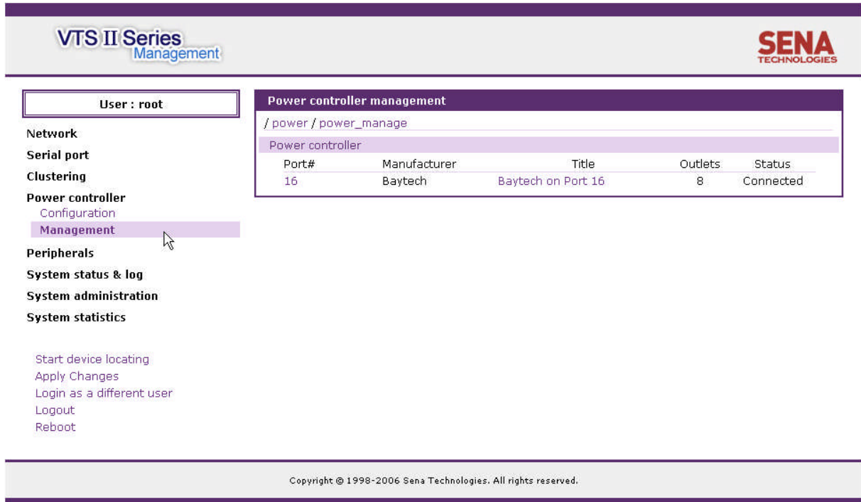
그림 6-7 파워 컨트롤러 관리 - 파워 컨트롤러 리스트
