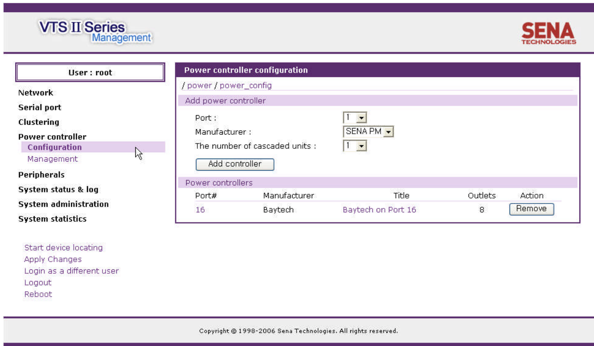
그림 6-1 파워 컨트롤러 설정
