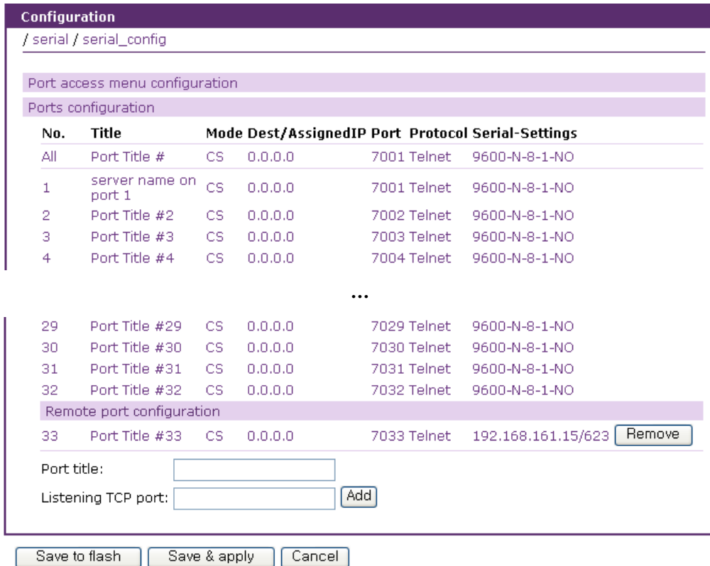
그림 4-1 시리얼 포트 설정 메인 화면
