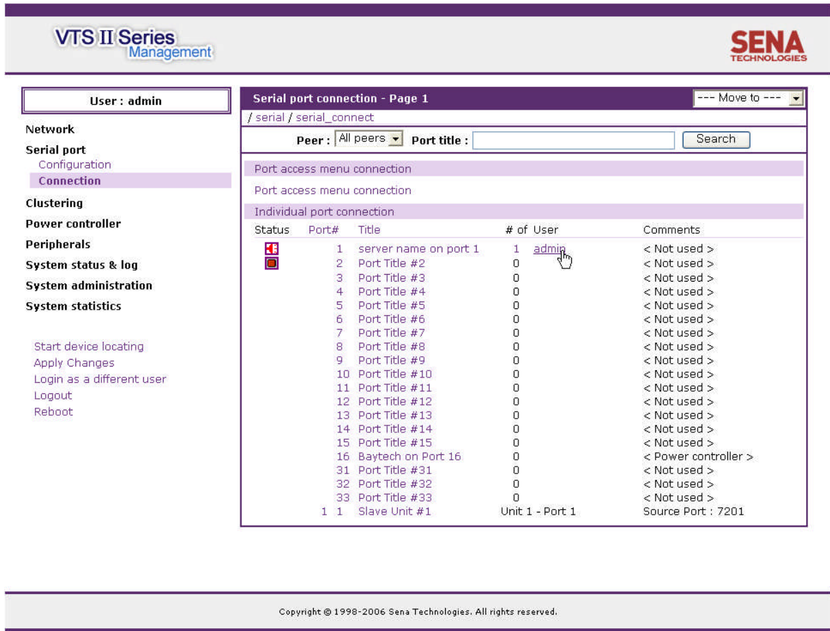
그림 4-31 시리얼 포트 연결 페이지
