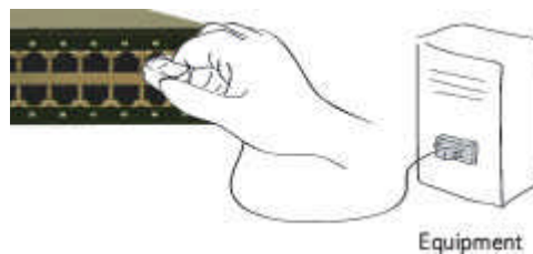
그림 2-5 장비를 VTS II에 연결하기
