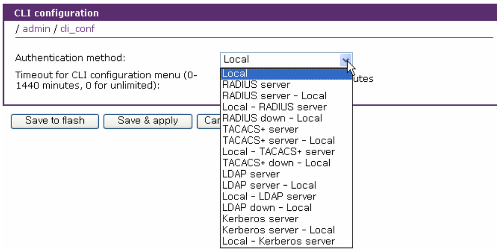
그림 9-16. CLI 설정
